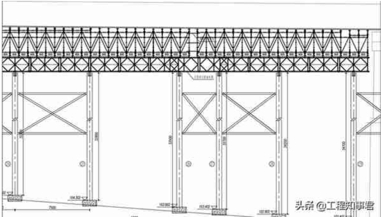
支架设计纵断面
